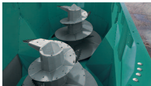
Préparation minutieuse : vis et couteaux préservant la structure du fourrage
