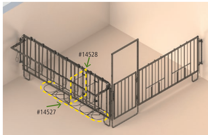
Rozwiązanie narożne szerokie: 2 x 14495 (uchwyt ścienny), 1 x 14496 (przęsło z drzwiami, długie) 1 x 14498 (krata ochronna, 7 stanowisk do karmienia)
