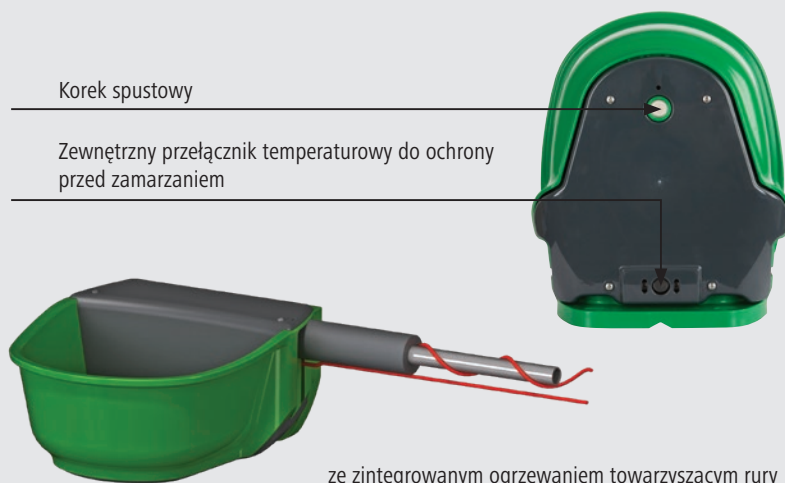
ze zintegrowanym ogrzewaniem towarzyszącym rury
