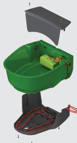
Ostona na spodzie poidła zapobiega uciekaniu ciepła oddawanego przez przewód grzewczy.
