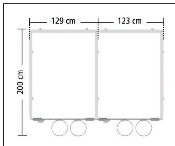
dimensiones exteriores: A = 200 cm, B = 129 cm, C = 123 cm
