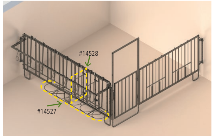
solución de esquina ancha: 2x 14495 (soporte de pared), 1x 14496 (pieza de cerca con puerta larga), 1x 14498 (cornadiza con 7 plazas de alimentación)
