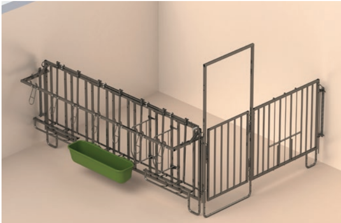
solución de esquina estrecha: 2x 14495 (soporte de pared), 1x 14491 (pieza de cerca con puerta corta), 1x 14498 (cornadiza con 7 plazas de alimentación)
