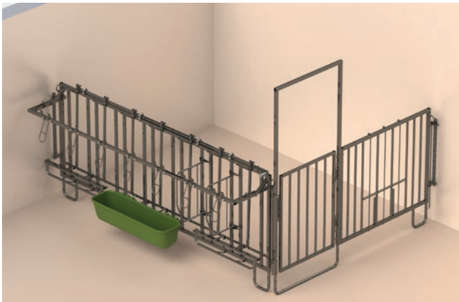
Hoekoplossing smal: 2 x 14495 (wandhouder), 1 x 14491 (afrasteringsgedeelte met deur kort), 1 x 14498 (vangrooster 7 plaatsen)
