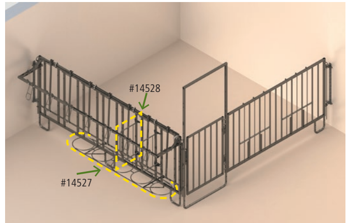
Hoekoplossing breed: 2 x 14495 (wandhouder), 1 x 14496 (afrasteringsgedeelte met deur lang), 1 x 14498 (vangrooster 7 plaatsen)
