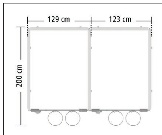
buitenmaten: A = 200 cm, B = 129 cm, C = 123 cm
