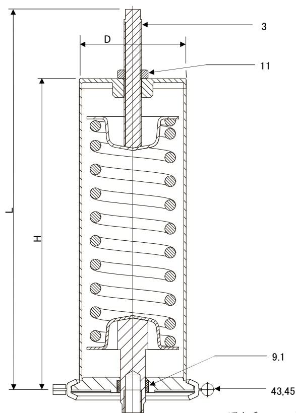
アクチュエーターF
