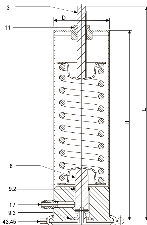
アクチュエーターF-CJ
