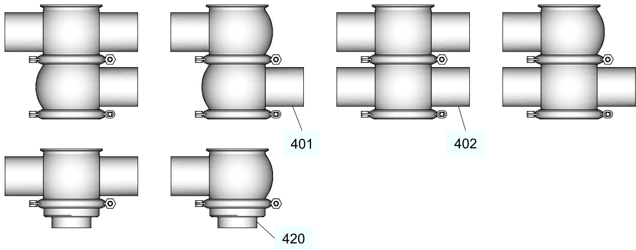
Abb.3: Gehäusekombinationen
