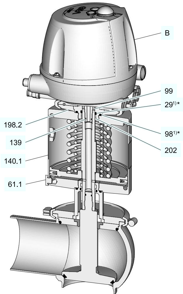
Fig.3: Avec tête de commande T.VIS
