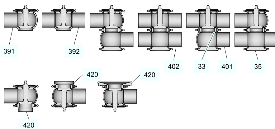
Fig.2: Combinaisons de boîtiers
