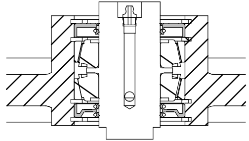
Installation des joints d'étanchéité
