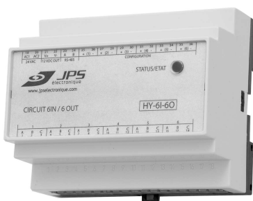
I/O MODULE 2005-2901-730
